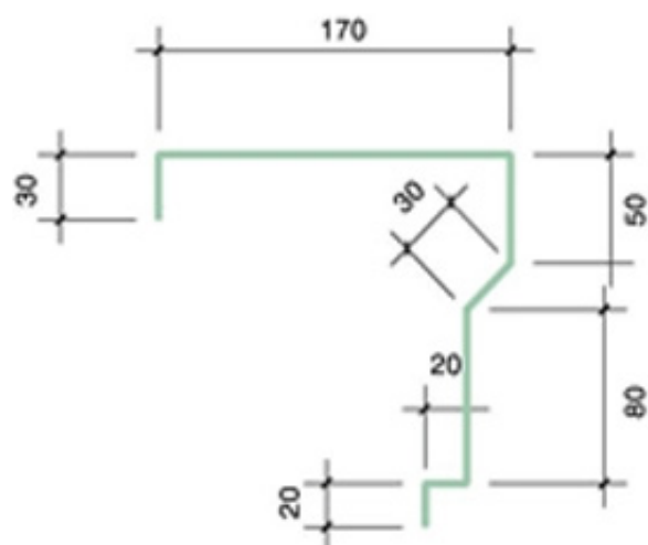
VIỀN MÁI GABLE TRIM
